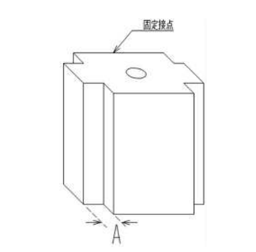
図3:固定接点
