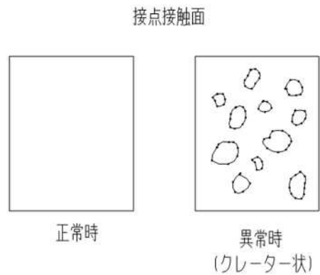
図2:接点状態
