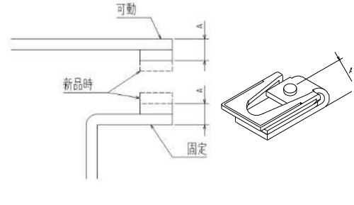
図3:接点厚み
