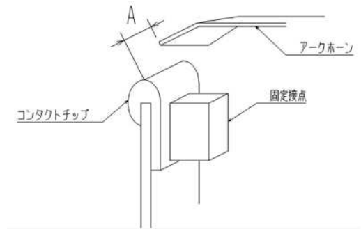
図3: 固定接点
