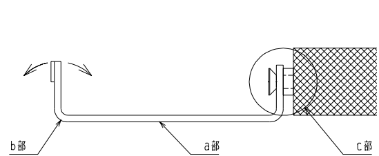
図6:補助固定接点
