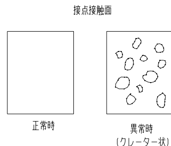
図2:接点状態
