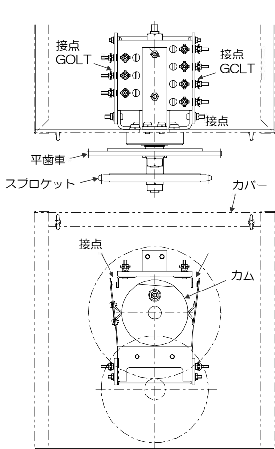
YA007A087 形 かごの戸全開感知スイッチ
