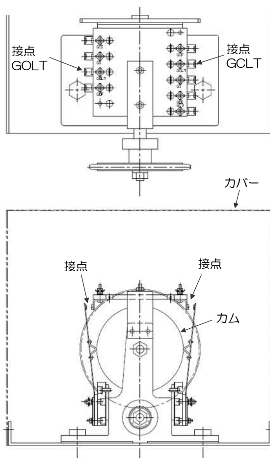
EL-2358 形、EL-8829 形 かごの戸全開感知スイッチ
