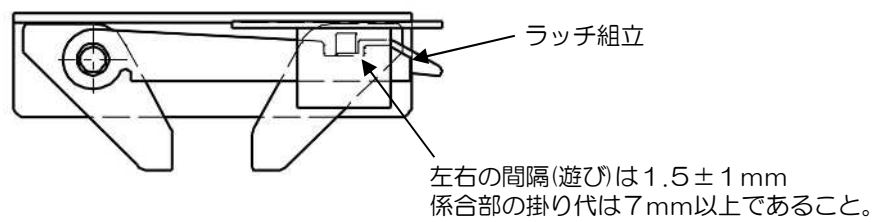
IL-11A形 乗場の戸スイッチ
