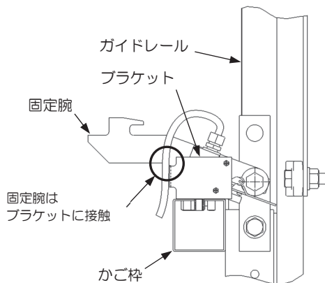
固定腕 収納状態
