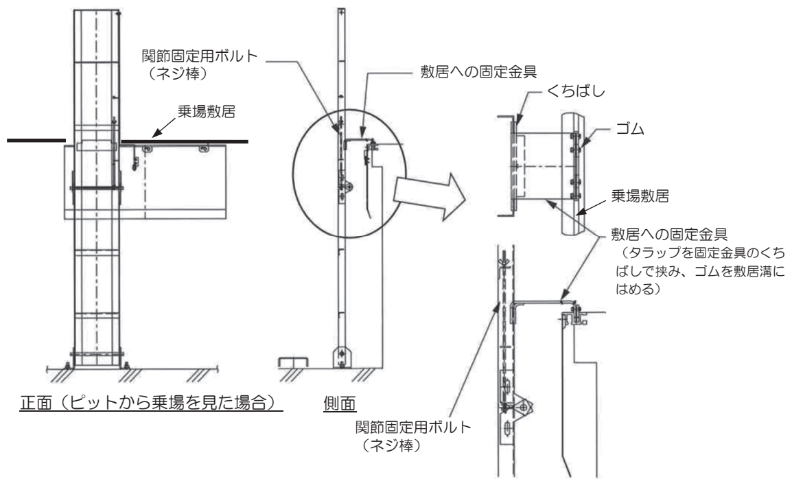
図 6.2(b) 折り畳み式ピットトラップ 組立状態
