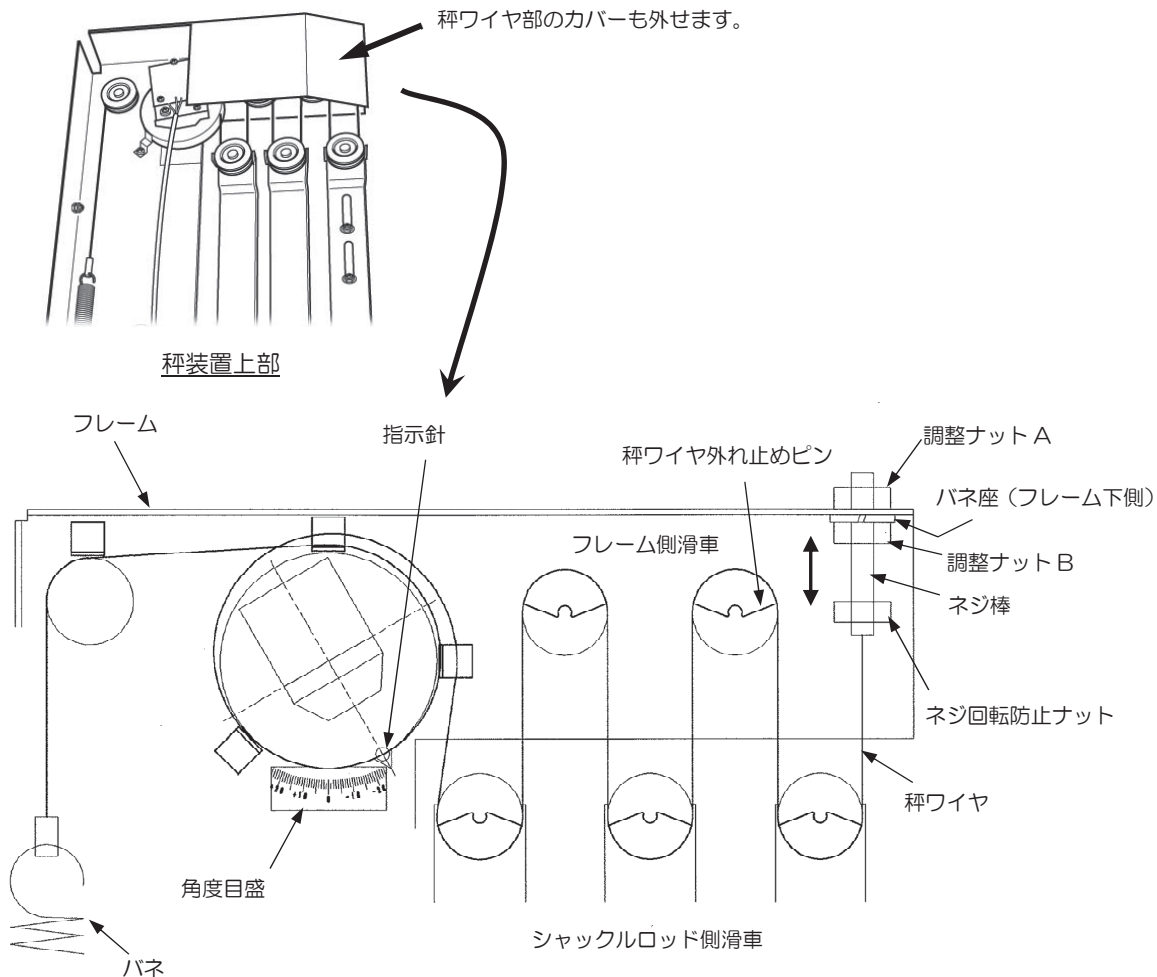
秤装置上部詳細図 (カバーを外した状態)
