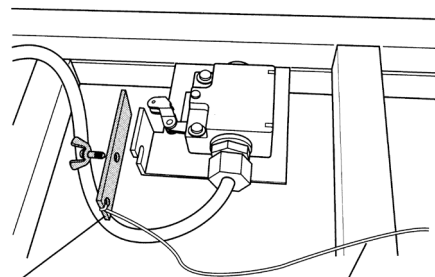
押え板
